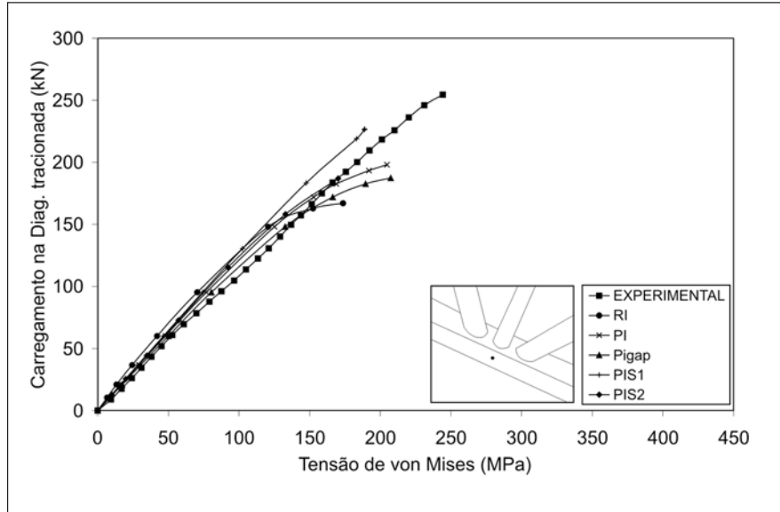
Figura 9 - Protótipo N8 (Roseta 3).
