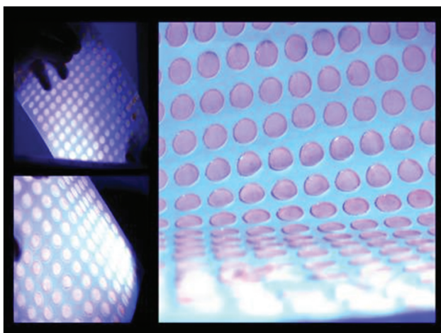
Figura 5. Sensores de radiação azul, baseados em MEH-PPV/Alq 3 /OS, fabricados em escala piloto. A figura mostra a foto de cerca de 150 selos recém-fabricados excitados opticamente com luz azul.
