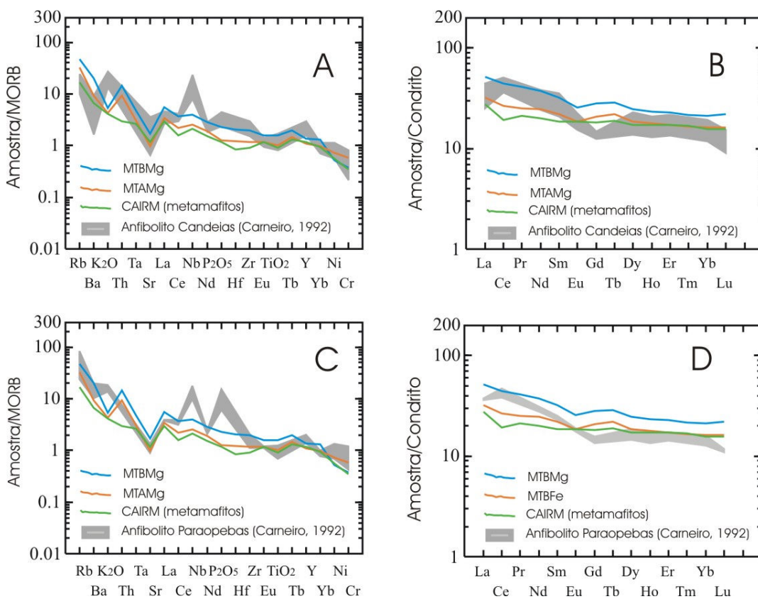
Figura 10.6 - Envelopes de variação de padrões geoquímicos dos anfibolitos Candeias e Paraopeba de Carneiro (1992), normalizados respectivamente ao MORB de Bevens et al. (1984) e ao condrito C1 de Boynton (1985), comparados às médias dos metamafitos estudados (linhas coloridas).
