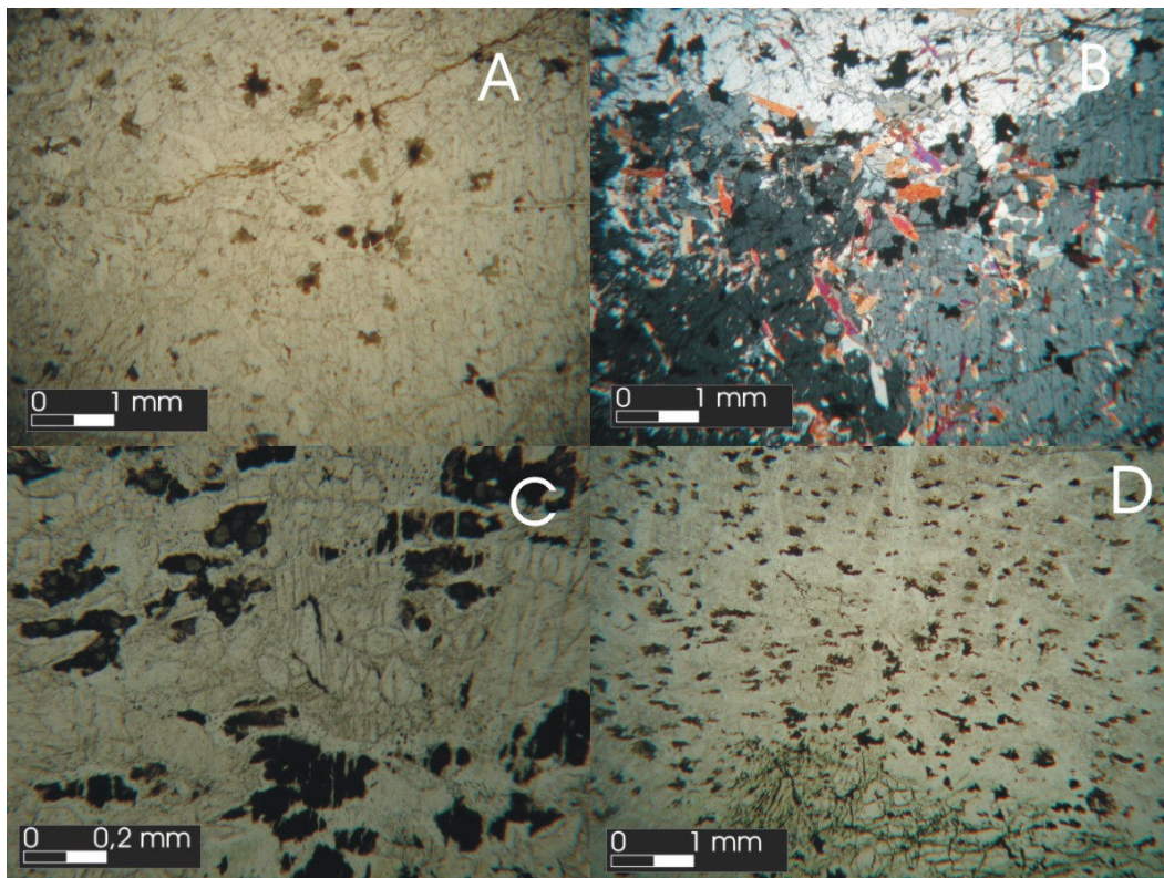
Figura 5.4 – A) Seção em metaortopiroxenito vista com polarizador descruzado. Nota-se a presença de cristais de espinélio disseminados (objetiva: 1.6x; pol.: //). B) Seção anterior vista com luz polarizada. Note-se o aspecto pegmatóide dos cristais de ortopiroxênio com anfíbolitização incipiente concentrada tanto nas bordas dos cristais quanto em seu interior. C) Cristais de espinélio e opacos exibindo estrutura pull-apart (objetiva:10x; pol.: //). D) Seção de metaortopiroxenito com espinélio e opacos disseminados (objetiva:1.6x; pol.: //).
