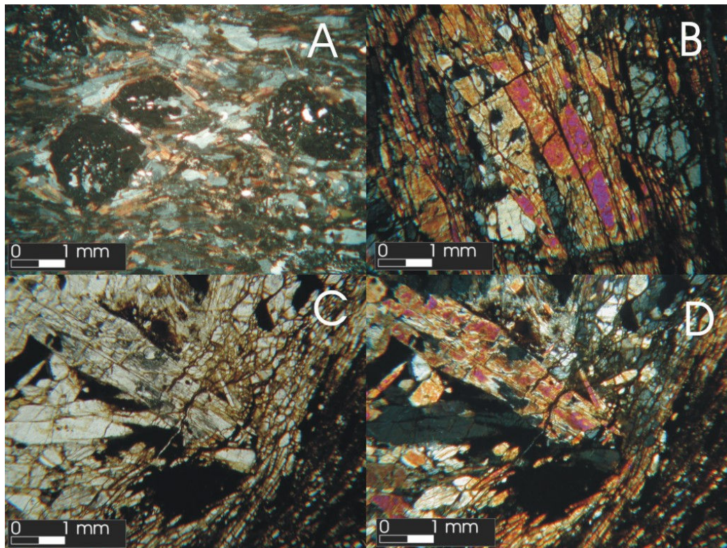
Figura 4.7 – A) Seção típica de granada-biotita-plagioclásio-quartzo xisto mostrando porfiroblastos amendoados sin-deformacionais de granada (mineral isotrópo) em matriz granolepidoblástica (objetiva 1.6x; pol.: X). B) Seção em granada-quartzo-sillimanita xisto mostrando feixe paralelo de sillimanita prismática (objetiva 1.6x; pol.: X). C) Seção da mesma lâmina anterior mostrando arranjo decussado de sillimanita prismática (objetiva 1.6x; pol.: //). D) Mesma seção anterior vista com luz polarizada (objetiva 1.6x; pol. //).
