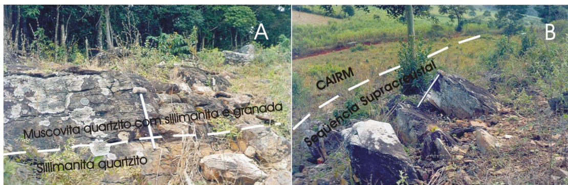
Figura 4.6 – A) Afloramento com intercalação de sillimanita quartzito e muscovita quartzito com sillimanita e granada, mostrado pela linha vermelha. B) Afloramento de sillimanita-quartzito em contato com o Complexo Acamadado Itaguara-Rio Manso, marcado pela linha vermelha.
