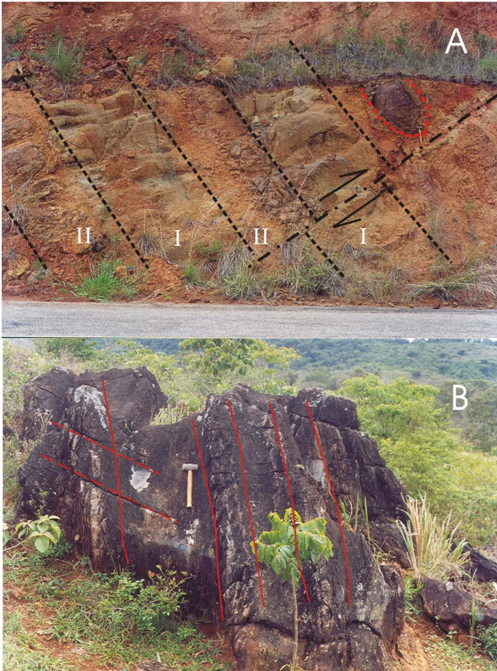
Figura 5.2 – A) Afloramento do ponto 54G176, mostrando em saprólito, acamamento magmático basculado e deslocado por zona de cisalhamento. Observa-se repetição cíclica das variedades litológicas em estratos com pouco mais de um metro de espessura, representada pelos algarismos romanos. Nota-se xenólito de ultramafito demarcado por linha vermelha tracejada. B) Acamamento magmático (linha vermelha contínua) cortado por foliação (linha vermelha tracejada).
