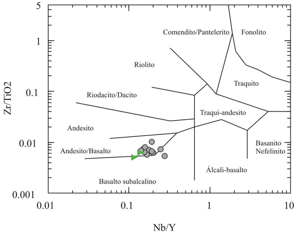
Figura 8.1 - Diagrama discriminante de rochas vulcânicas de Winchester & Floyd (1977). Círculos cinza: Unidade Metamáfica indiscriminada. Triângulos verdes: metamafitos do CAIRM.
