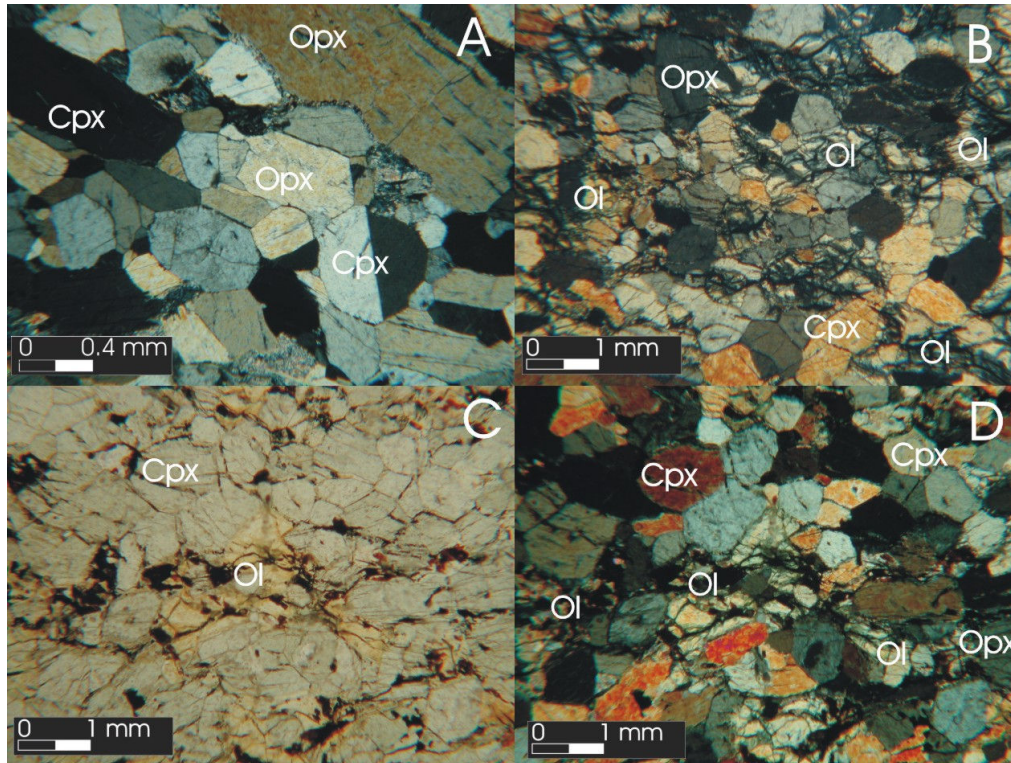
Figura 5.7 – A) Seção em metawebsterito obtido no ponto 54KJ49, mostrando textura adcumulática biminerálica a clino e ortopiroxênio (objetiva: 5x; pol. X). B) Seção em meta-olivina-websterito exibindo textura mesocumulática entre ortopiroxênio, clinopiroxênio e olivina. (objetiva: 1.6x; pol. X). C) Vista de outra região da lâmina anterior, analisada com polarizador des cruzado, exibindo textura adcumulática a orto e clinopiroxênio com olivina intercumulus . Nota-se olivina alterando-se para iddingsita (alteração marrom; objetiva 1.6x; pol. //). D) Seção anterior vista com polarizador cruzado.
