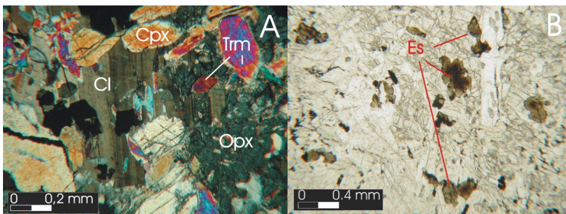
Figura 5.6 – A) Fotomicrografia de meta-olivina-ortopiroxenito obtida a partir de amostra do ponto 54GJ78, mostrando a presença de clinoclóro (Cl) e tremolita (Trm) entre os minerais secundários (objetiva de 10x, pol. X). B) Outra região da lâmina anterior mostrando espinélios (Es) marrons sobrecrecidos por espinélios esverdeados (objetiva de 5x, pol. //).
