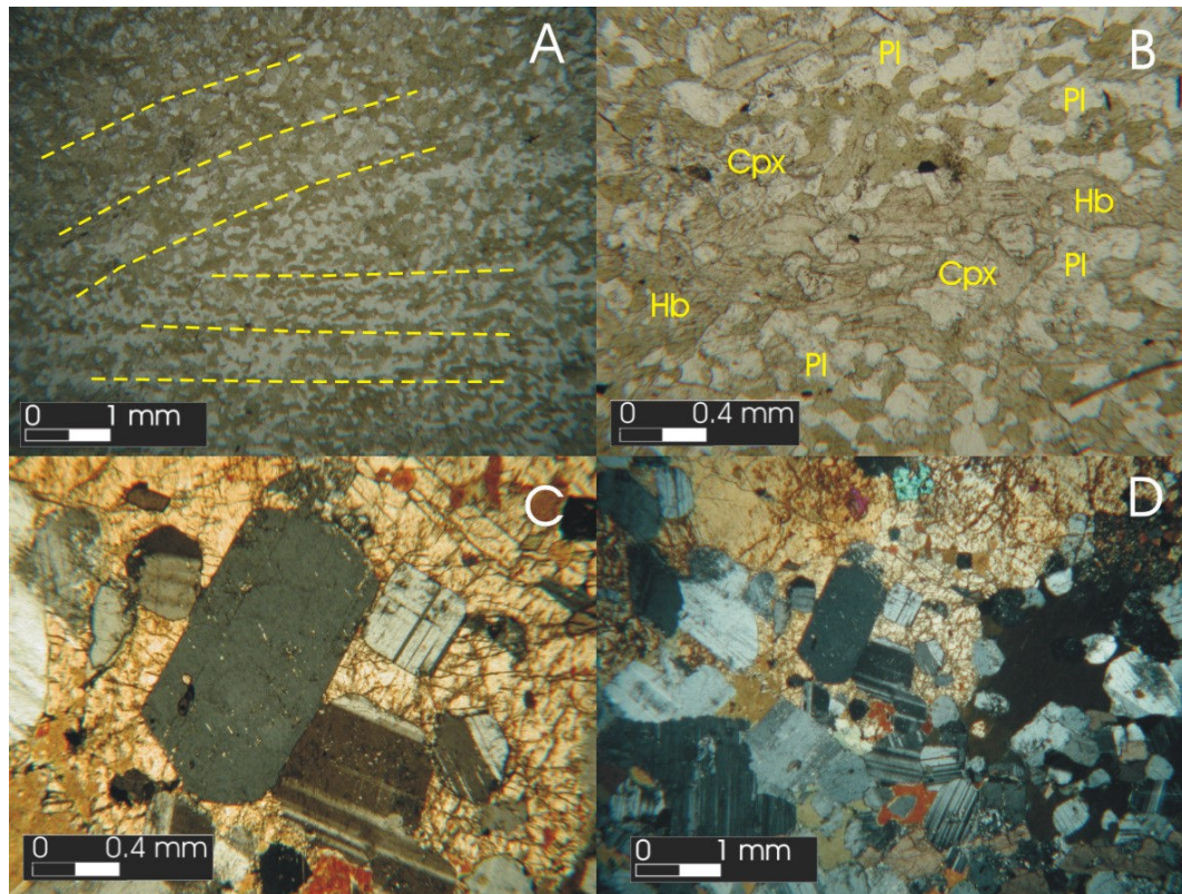
Figura 5.9 – A) Metagabro fino, obtido no ponto 54LH57. As linhas tracejadas mostram estratificação magmática em duas direções se cruzando. Os cristais de hornblenda cresceram sobre mesocumulosos a clinopiroxênio e plagioclásio (objetiva: 1.6x; pol. //). B) Vista em detalhe da seção anterior. Nota-se a presença de hornblenda que se desenvolveu sobre os microrritmos a partir anfibolitização do clinopiroxênio. (objetiva:5x; pol. //). C) Textura heteradumulática obtida em amostra do ponto 54HG63 caracterizada por cristais euédricos de plagioclásio englobados por megacristal de augita (objetiva: 5x; pol.: X). D) Vista anterior com aumento reduzido, mostrando graduação de textura adcumulática monomineralica a plagioclásio (base da Figura) para textura heteradumulática (topo da foto; objetiva: 1.6x; pol. X).
