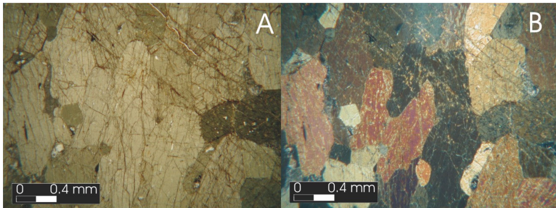
Figura 5.8 – A) A fotomicrografia apresenta textura adcumulática em hornblendito obtido no ponto 54KI41 (objetiva 5x; pol. : //). B): Seção anterior vista com luz polarizada (objetiva 5x; pol:X).
