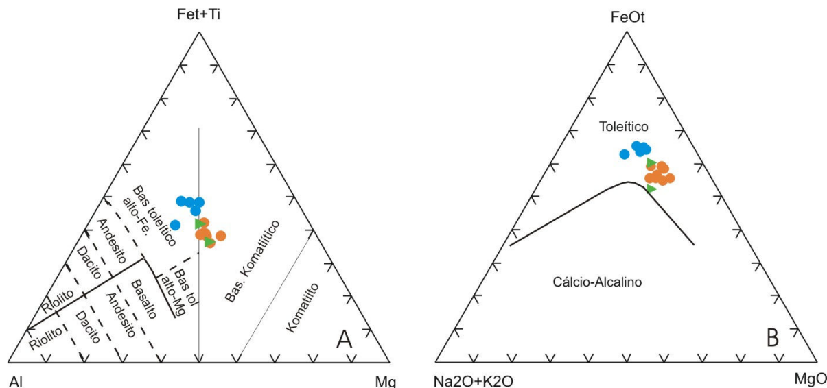
Figura 8.3 –A) Diagrama proposto por Jensen (1976, modificado por Rickwood 1989), para discriminação de suítes cálcio-alcálicas, tholeiíticas e komatiíticas. B) Diagrama AFM (álcalis totais – FeO – MgO) de Irvine & Baragar (1971), para classificação de rochas máficas mostrando uma variação de caráter tholeiítico a cálcio-alcálico. Círculos azuis: MTBMg; círculos laranjas: MTAMg; triângulos verdes: metamafitos do CAIRM.
