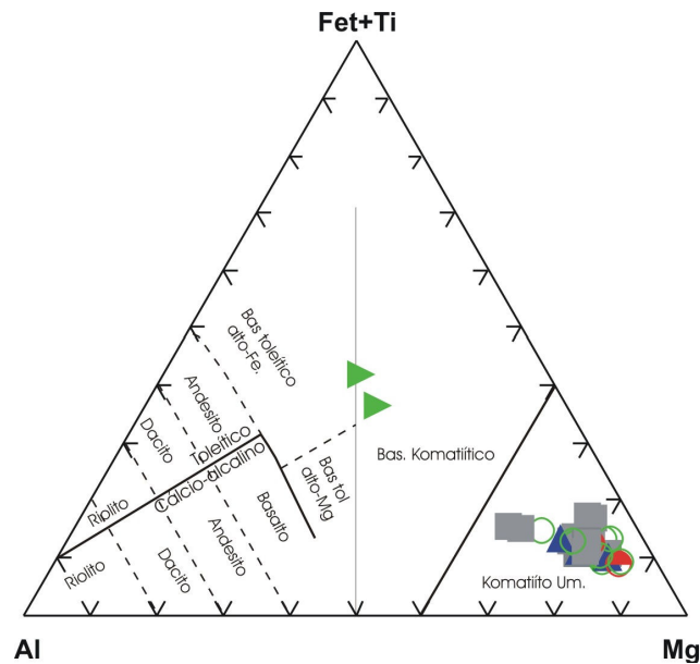
Figura 9.2 - Diagrama discriminante de Jensen (1976) (corrigido por Rickwood 1989), para komatiitos, tholeiitos e rochas cálcio-alcálicas. O diagrama utiliza a proporção catiônica dos elementos Al, Mg, Fe e Ti para discriminar os grupos litológicos a que se propõem. Convenções: como a figura anterior.
