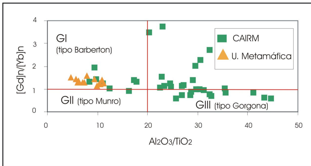
Figura 10.2 – Diagrama de Arndt (1994) segundo a proposta de Jahn et al. (1982) para classificação de suítes komatiíticas. O diagrama aqui apresentado tenta mostrar a evolução magmática a partir de uma tendência negativa entre as razões Al_2O_3/TiO_2 e [Gd]_n/[Yb]_n onde aparentemente as rochas plotadas transicionam de komatiítos do tipo Gorgona para Komatiítos do tipo Barberton. Nesse caso, os metatholeiítos da Unidade Metamáfica são plotados meramente com a finalidade de comparação. As linhas indicam os valores condríticos.
