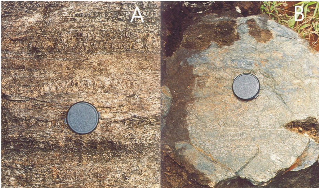
Figura 5.3 – A) Detalhe de microestratificações (microrítmos). B) Textura cumulática em metaharzburgito.
