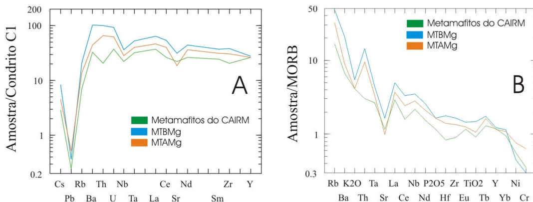
Figura 8.6 - Diagramas multi-elementares dos metamafitos da Seqüência Supracrustal. Para fins de comparação, também estão plotados no diagrama os metamafitos encontrados no CAIRM. Normalização: MORB (Bevins et al. 1984) e Condrito C1 (Sun & McDonough 1989).
