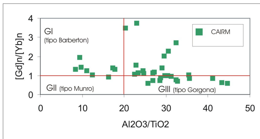
Figura 9.3 - Diagrama adaptado de Arndt (1994) apresentando a classificação de rochas ultramáficas komatiíticas propostas por Jahn et al. (1982). As linhas representam valores condríticos. As razões [Gd]_n/[Yb]_n foram normalizadas como os valores de manto primitivo de Sun & McDonough (1989), embora no trabalho original tivessem sido adotados os valores do manto primitivo de Hofmann (1988).
