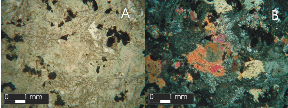
Figura 6.3 – A) Seção de gabro típico do SDM-NE (objetiva: 1.6x; pol. //). B) Vista anterior com luz polarizada. Observa-se vestígios de textura subofítica, superimosta por avançado metamorfismo de baixo grau (objetiva: 1.6x; pol. X).
