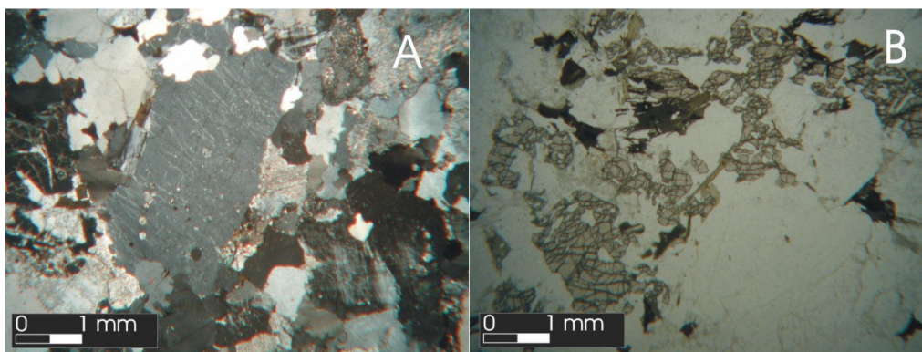
Figura 6.5 – A) Detalhe de textura porfiróide com k-feldspato pertítico (objetiva 1.6x; pol. X). B) Fenocristais de granada configurando a textura porfírica (objetiva 1.6x; pol. //).
