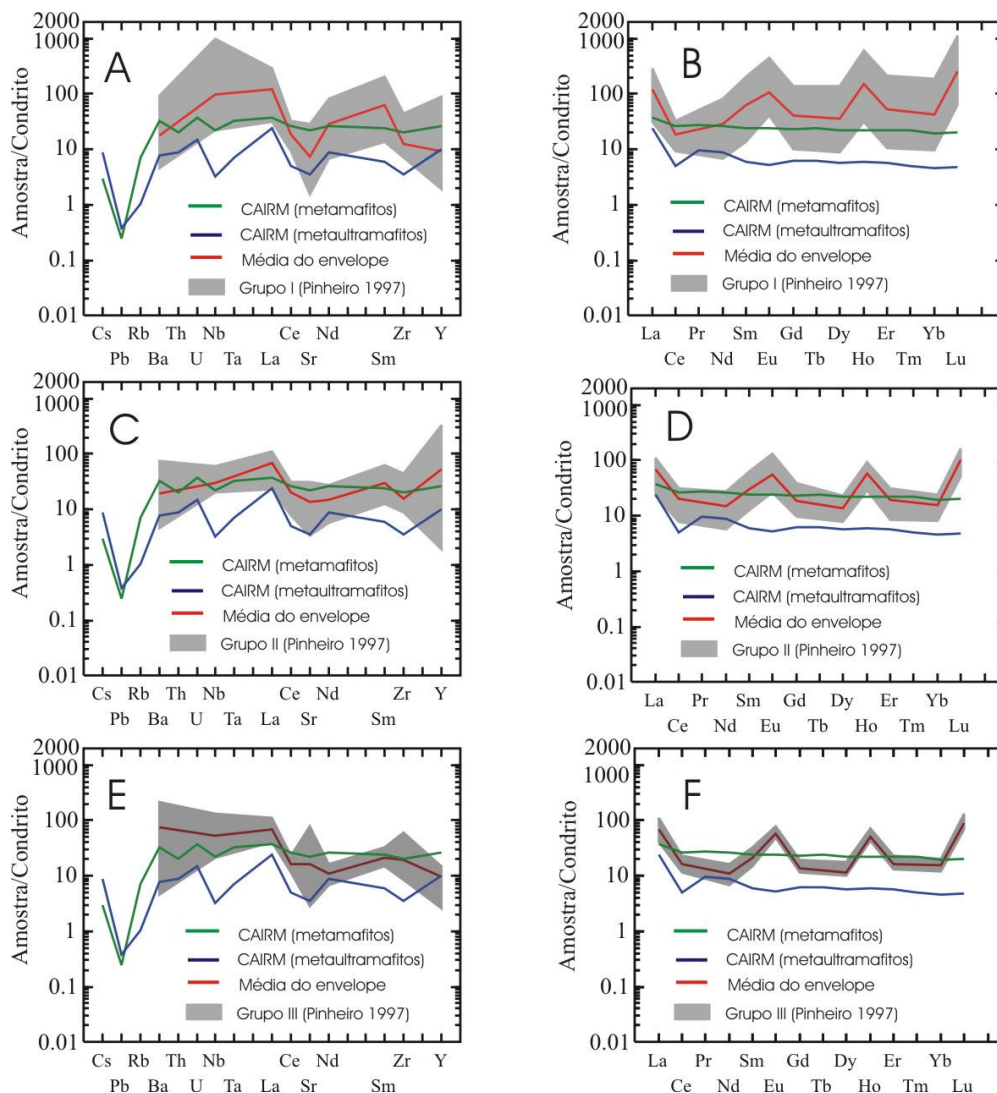
Figura 10.10 - Envelopes de variação de padrões geoquímicos dos komatiitos dos Grupos I, II, III, definidos por Pinheiro (1998) na região do Morro da Onça, Rio Manso/Mg, normalizados ao condrito C1 de Sun & McDonough. (1989) e comparados às médias das amostras do CAIRM (linhas coloridas).
