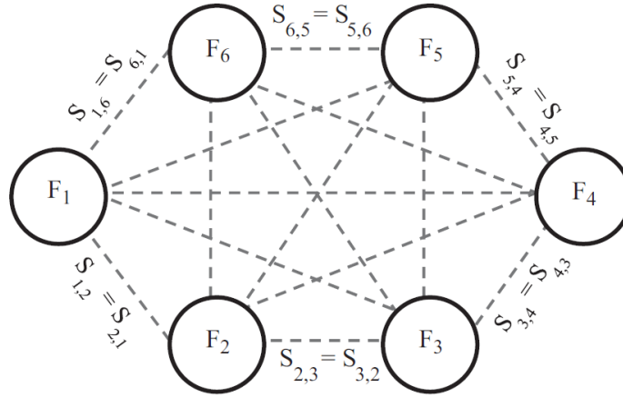
Figura 3.1: Representação gráfica de um problema de Seleção de Atributos onde S_{i,j} representa a similaridade associada a cada nó entre as variáveis i e j . Em outras palavras, S_{i,j} = sim(F_i, F_j) . Fonte: Tabakhi et al. (2014).
