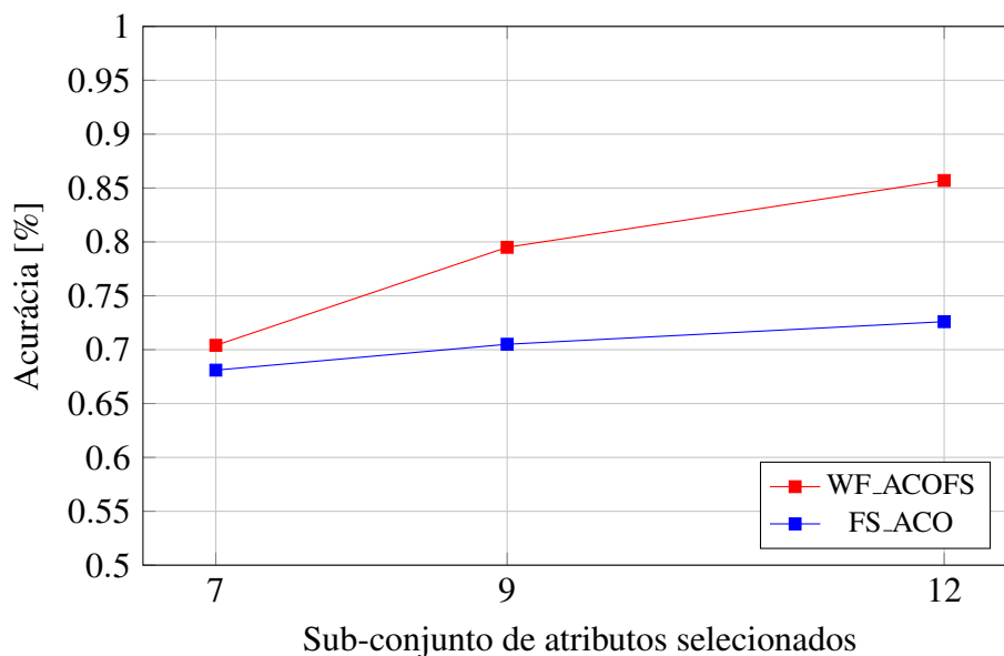
Gráfico 4.2: Valores da Média de Acurácia %, após 10 execuções, obtidos através da classificação KNN para o banco de dados Lymprografy :
