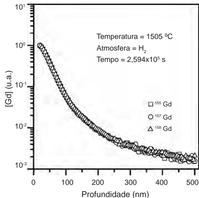
Figura 3: Curvas de penetração normalizadas dos isótopos ^{155}\text{Gd} , ^{157}\text{Gd} e ^{158}\text{Gd} no \text{UO}_2 policristalino.
