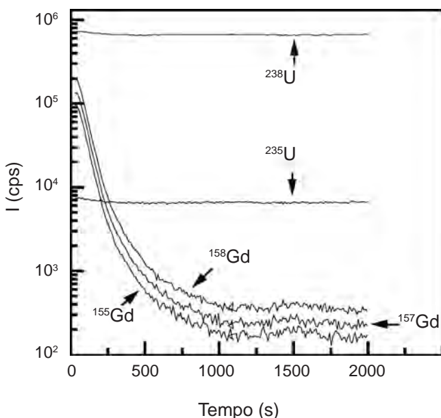
Figura 2: Espectro SIMS típico após difusão dos isótopos do gadolínio a 1505\ ^\circ\text{C} , durante 72 h. [Figure 2: Typical SIMS spectrum after diffusion of the Gd isotopes at 1505\ ^\circ\text{C} for 72 h.]
