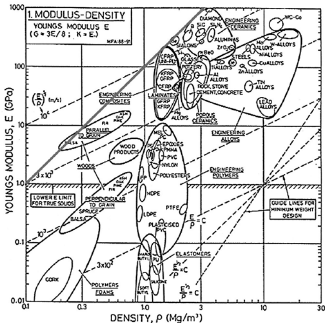
Figura 5 • Mapa de Ashby. Neste mapa de Ashby, cruzam-se todas as famílias de materiais quanto à resistência, à elasticidade em relação à densidade. A linha vermelha liga os materiais com o menor peso possível para uma performance que requeira resistências entre 1 e 1000 GPa. A 10 GPa, a madeira balsa seria escolhida (fibras paralelas); a ± 100 GPa, compósitos reforçados por fibras; a ± 1000 GPa, nem mesmo o diamante serviria. Numa segunda rodada, por exemplo, poderia ser definida uma faixa mais estreita de resistência versus custos máximos e seria admitida uma maior densidade (mais peso). Fonte: ASHBY; JONES, 1980.
